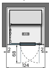
WNĘKA W
