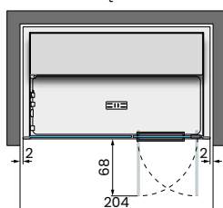
WNĘKA W
