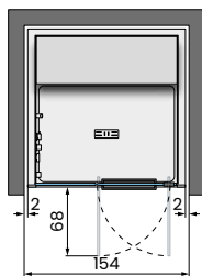
WNĘKA W
