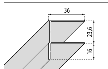
VERBREDINGSPROFIEL +10 mm PROFILÉ D'ÉLARGISSEMENT +10 mm
