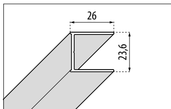
MUURPROFIEL PROFILE MURAL
