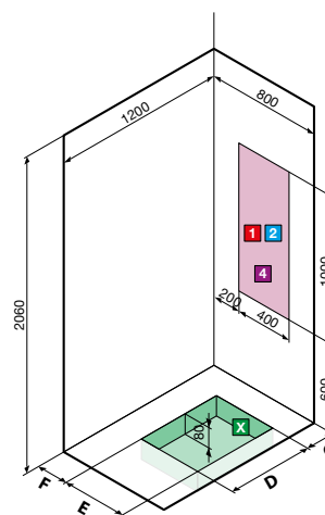
versione destra
