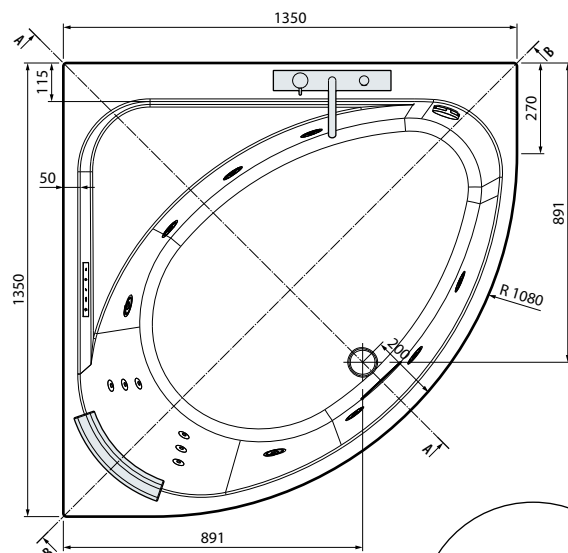
PARTICOLARE VASCA AD INCASSO
