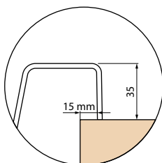
PARTICOLARE VASCA AD INCASSO
