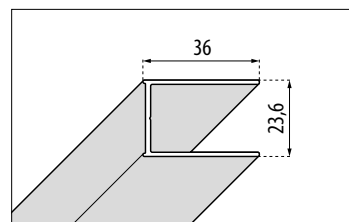
COMPENSAZIONE +10 mm
