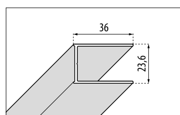
COMPENSADORES +10 mm
