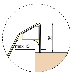
DETALLE DE BAÑERA EMPOTRADA
