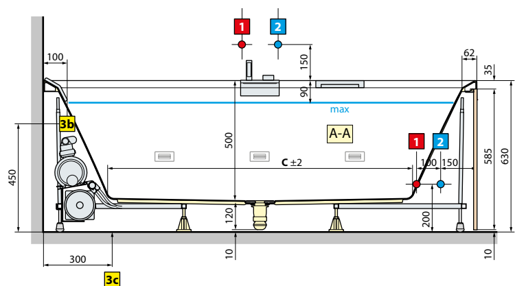
DETALLE DE BAÑERA EMPOTRADA
