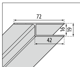
Standard Profil seitliche Wandmontage für alle Modelle
