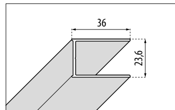
VERBREITERUNG +10 mm
