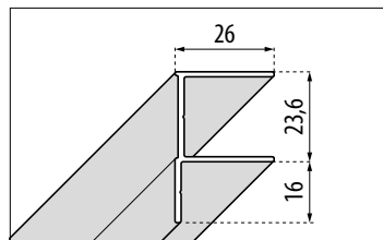
STANDARD PROFIL
