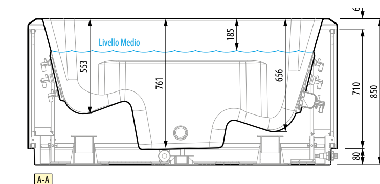
A-A
