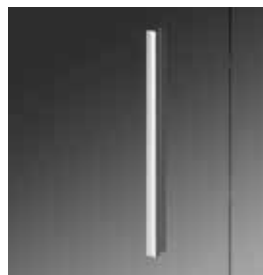
Uchwyt (do drzwi przesuwnych) Rozstaw osi 256 mm
