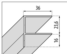
VERBREDINGSPROFIEL PROFILÉ D'ÉLARGISSEMENT +10 mm
