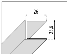
MUURPROFIEL PROFILÉ MURAL
