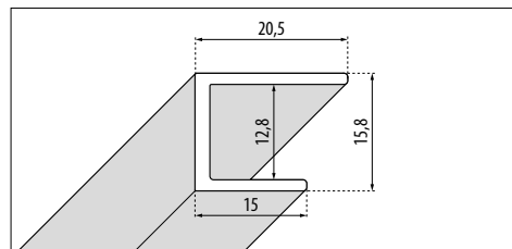
PRZYŚCIENNY - Wysokość 1998 mm dla N180 1B - strona magnesu
