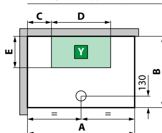
S WERSJA LEWA
