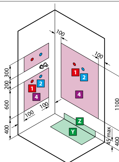
Wersja lewa Dla modeli A90x70 - A100x70 - A100x80 - 2P120x80
