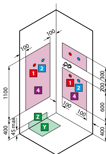
Dla modeli A80 - A90 - R90 - GF80 - GF90
