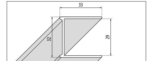
MUURPROFIEL ZIJWAND PROFILÉ MURAL PAROI LATÉRALE N180 GFL
