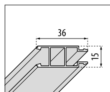
Verbreiterungsprofil für alle Modelle
