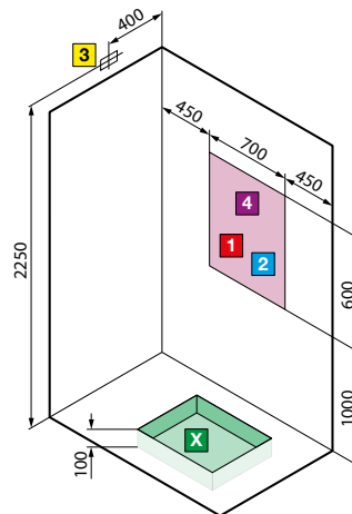
Links/Rechts für Eckmontage
