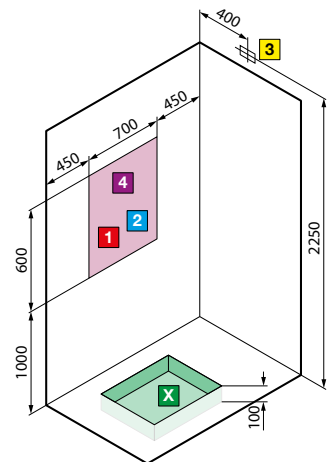
Links/Rechts für Eckmontage
