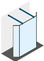
KUADRA FC + KUADRA HA x2 STABILISATIONSSTANGE (im Lieferumfang)
