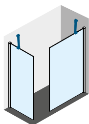
GIADA H x2 VERSTELLBARE STABILISATIONSSTANGE
