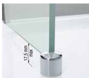
AUSGLEICHSHALTERUNG FÜR MONTAGE AUF BRAUSETASSE TEIL HL Ø 29 MM
