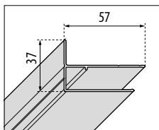
Verbreiterungsprofil 2P - G - B - S2 - 3P - 2A
