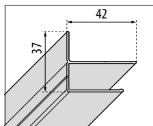
Standard Profil 2P - G - B - S2 - 3P - 2A
