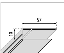
Verbreiterungsprofil A - R - F - AH - PH - FH
