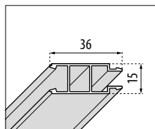
Verbreiterungsprofil für alle Modelle
