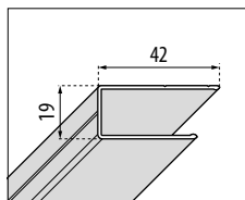
Standard Profil A - R - F - AH - PH - FH
