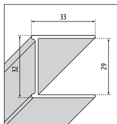
A MURO per Opera FH
