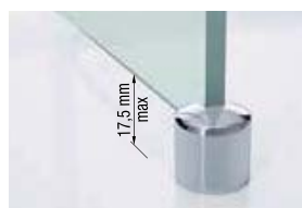
PIEDINO DI FISSAGGIO INTERNO AL PIATTO DOCCIA Ø 29 MM
