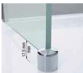
PIEDINO DI FISSAGGIO INTERNO AL PIATTO DOCCIA Ø 29 MM
