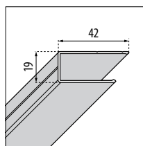
PROFILÉ DE SÉRIE A - R - F
