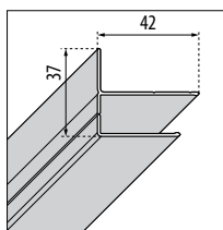
PROFILÉ DE SÉRIE 2P - G - B - S - S2 - 3P - 2A
