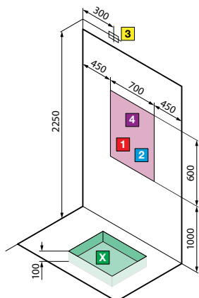
Installation au centre du mur
