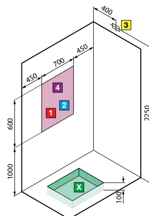
installation en angle
