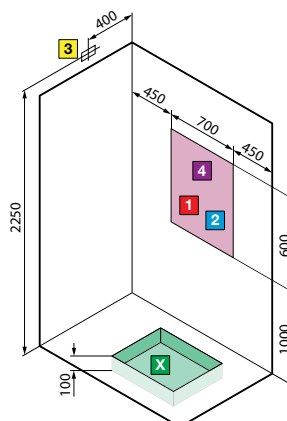
installation en angle
