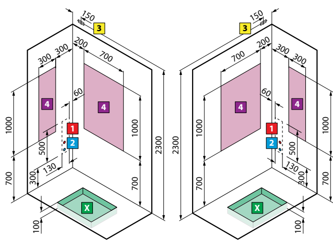
installation à gauche installation à droite modèles 2P140x80 - 2P140x90
