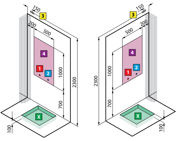
installation à gauche installation à droite A100x80 modèles A100x80 - 2P120x80
