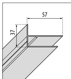
Verbreiterungsprofil G+FL - 3P - S - B - G
