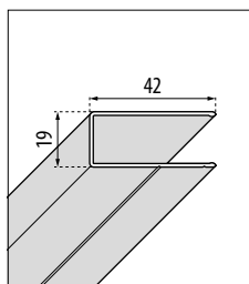
Standard Profil R - 2A - 2P - 2PH A - AH - 3PH
