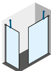
KUADRA H x2 VERSTELLBARE STABILISATIONSSTANGE
