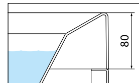
WANNENRAND - 8 CM
