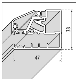
Mauerprofil für alle Modelle
