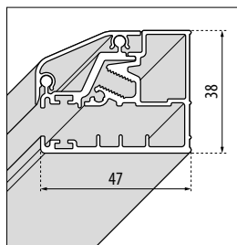
Mauerprofil für alle Modelle
