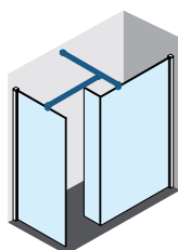
KUADRA H x2 KUADRA HL Drażek (w zestawie)
