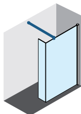
GIADA H GIADA HL STANDARD DRAŻEK STABILIZACYJNY (w zestawie)
