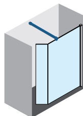
GIADA H GIADA HFA STANDARD DRAŻEK STABILIZACYJNY (w zestawie)
