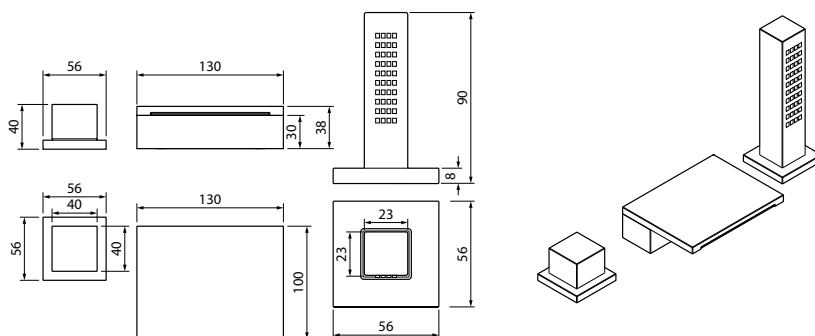
BATERIA WANNOWA TRÓJOTWOROWA (z przełącznikiem na wylewkę wannową lub słuchawkę prysznicową)
