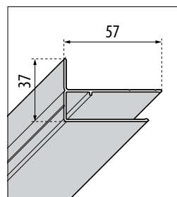
EXTENSION G+FL - 3P - S - B - G
