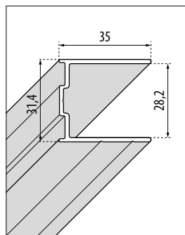
WALL - FREE 3
