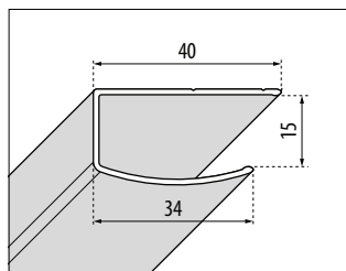
WALL - FREE 2
